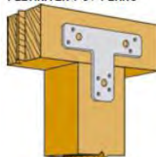
PLETINA EN T C / PERNO
