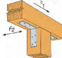
ANGULO DE REFUERZO
