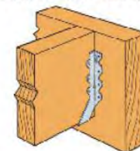
SOPORTE DE VIGA M / CEPILLADA
